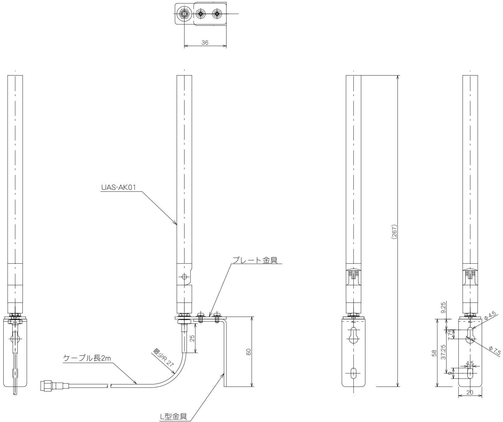
UAS-PK02 プレート付アンテナ外觀寸法図
